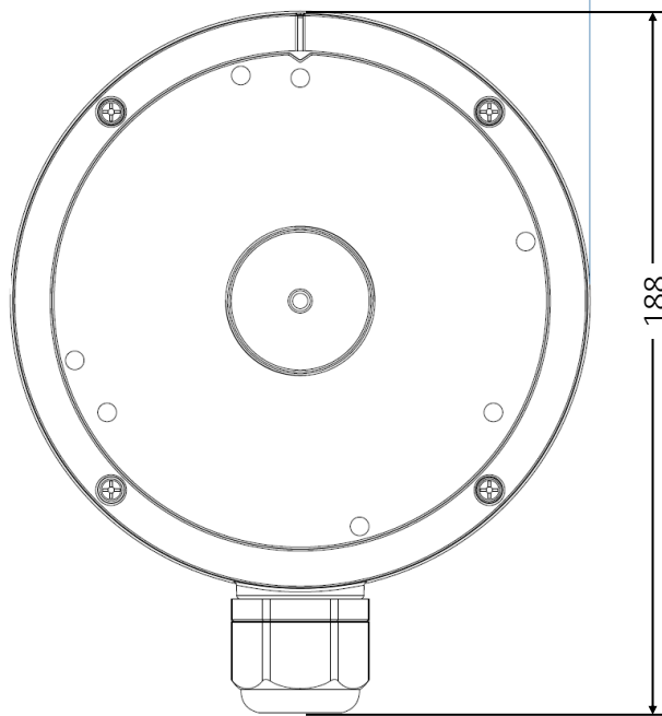
Top view for NVB-6040JB Widok z góry dla NVB-6040JB
