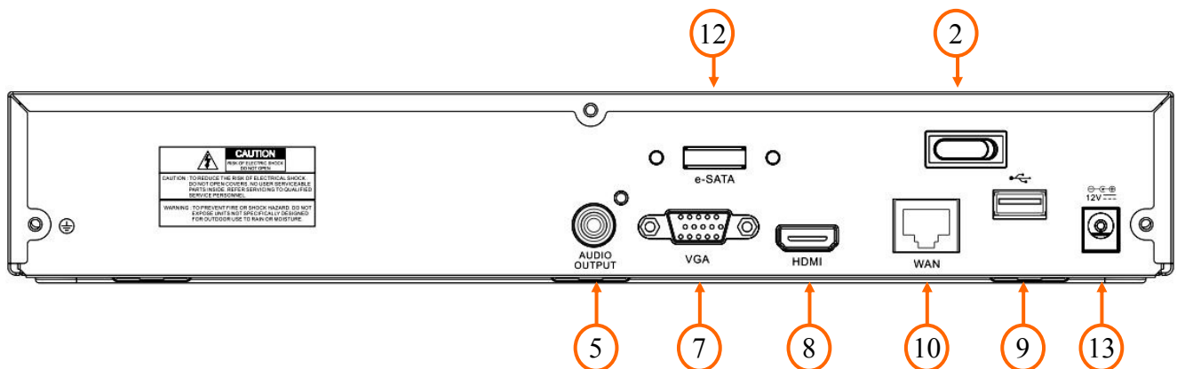
NVR-4116-H1
