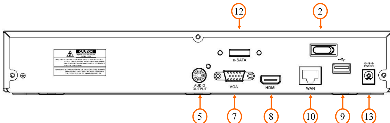
NVR-4116-H1
